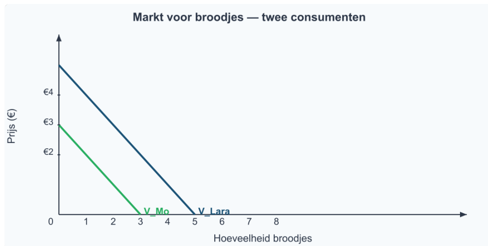
Figuur 8: Markt voor broodjes — V_Lara en V_Mo
